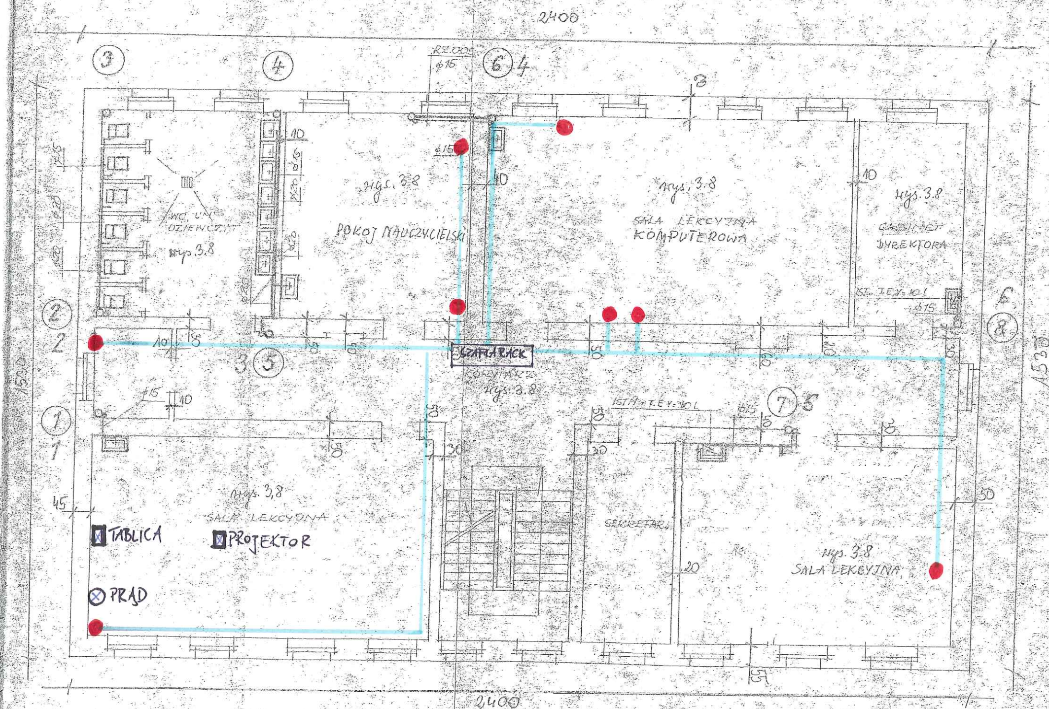
RZUT I PIĘTRA SKALA 1:100
